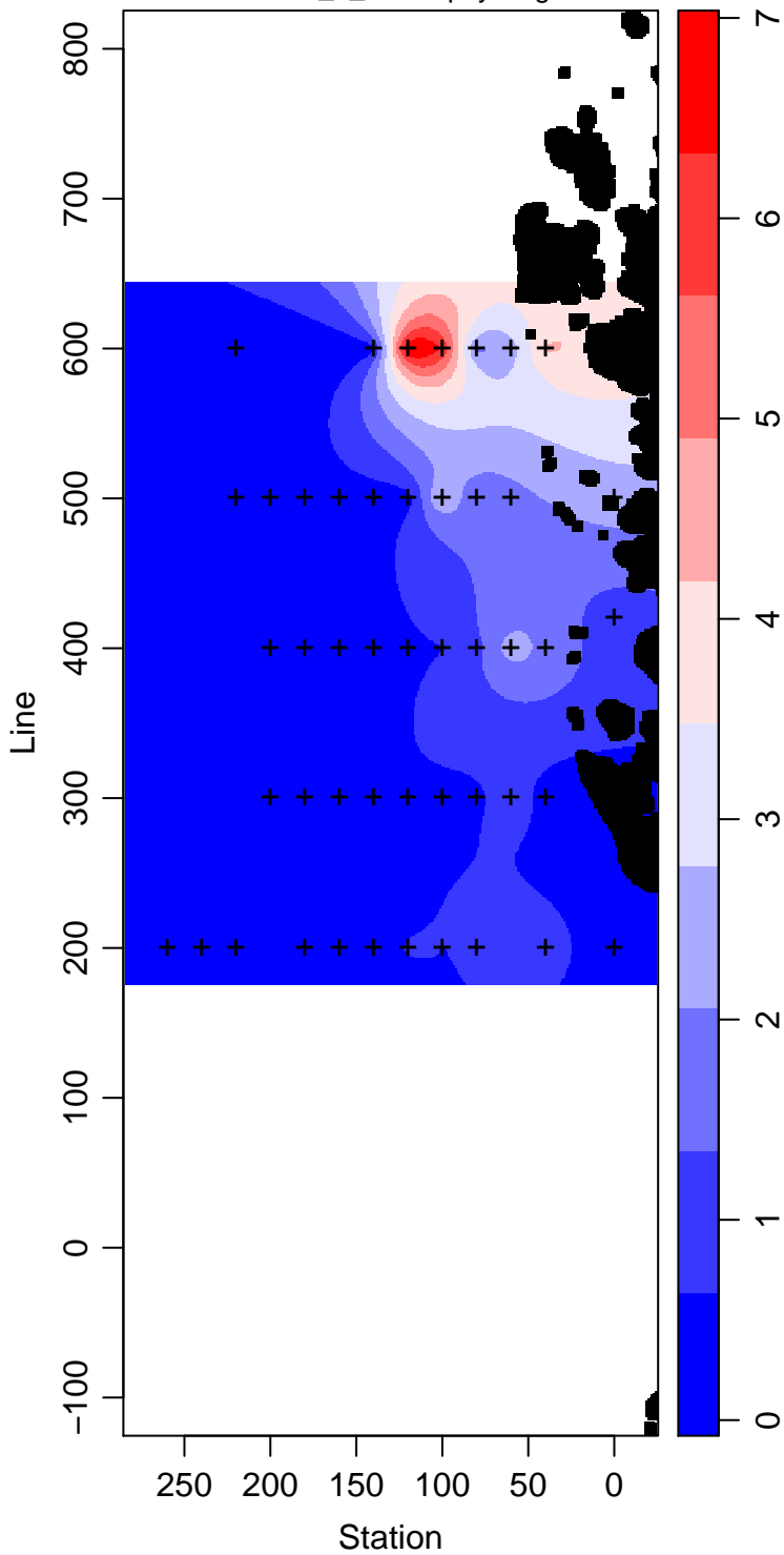
LMG08-01_1_Chlorophyll mg m -3
