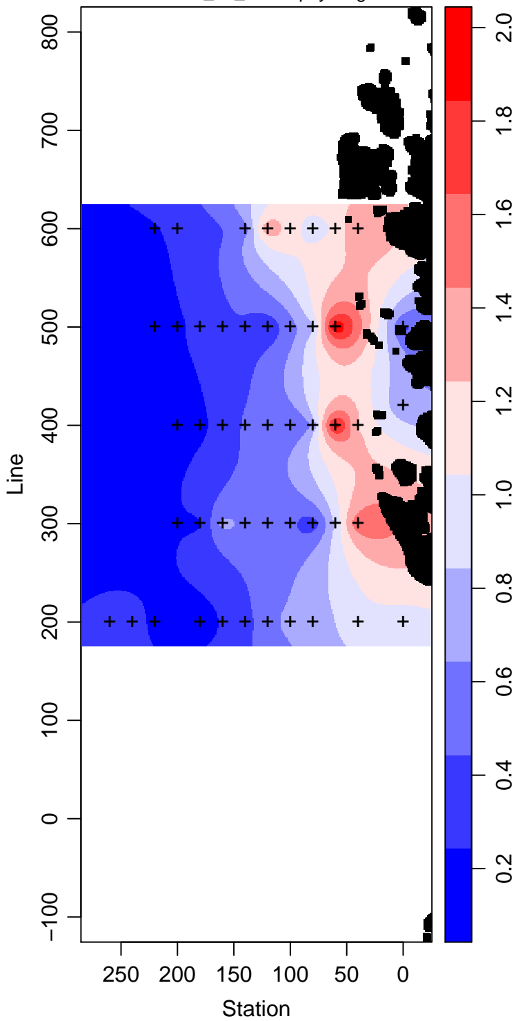
LMG08-01_20_Chlorophyll mg m -3
