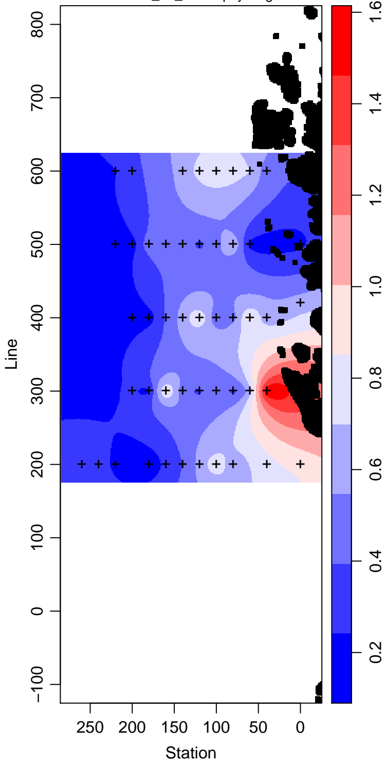
LMG08-01_35_Chlorophyll mg m -3
