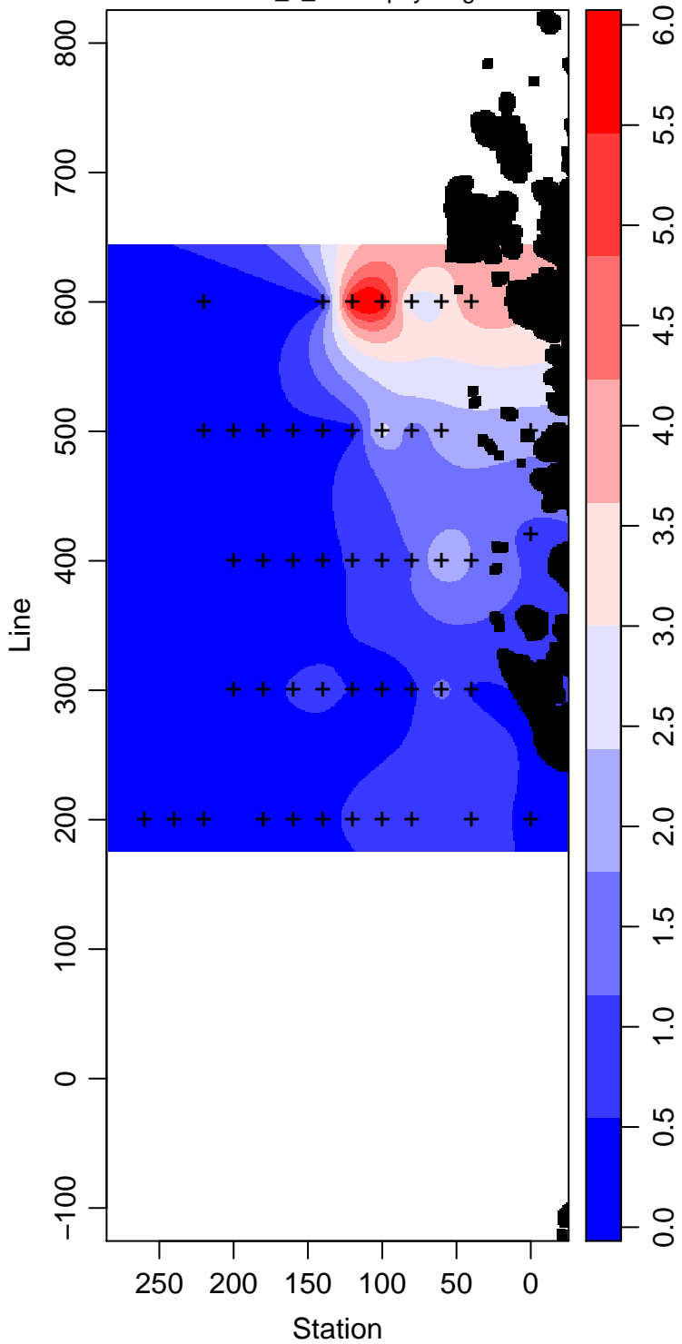
LMG08-01_5_Chlorophyll mg m -3
