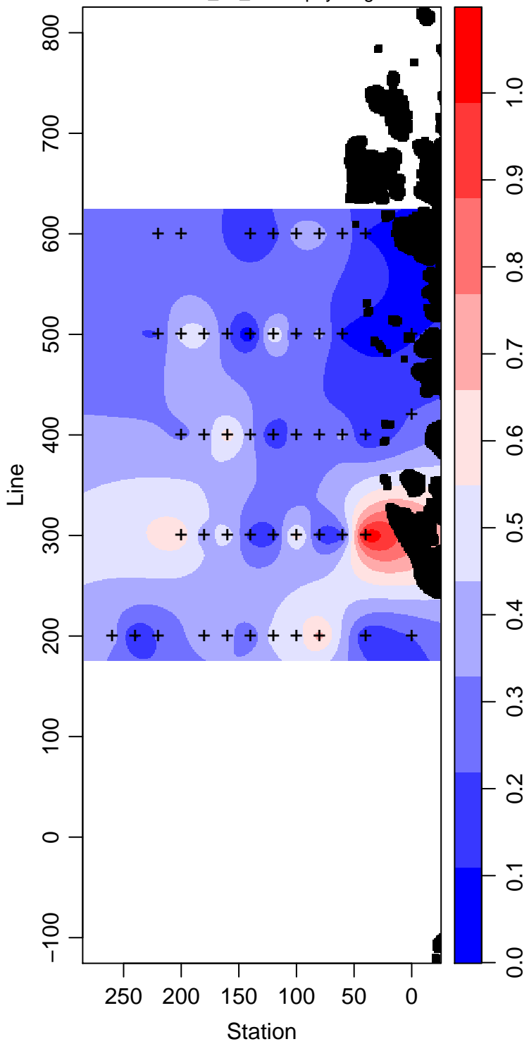
LMG08-01_65_Chlorophyll mg m -3
