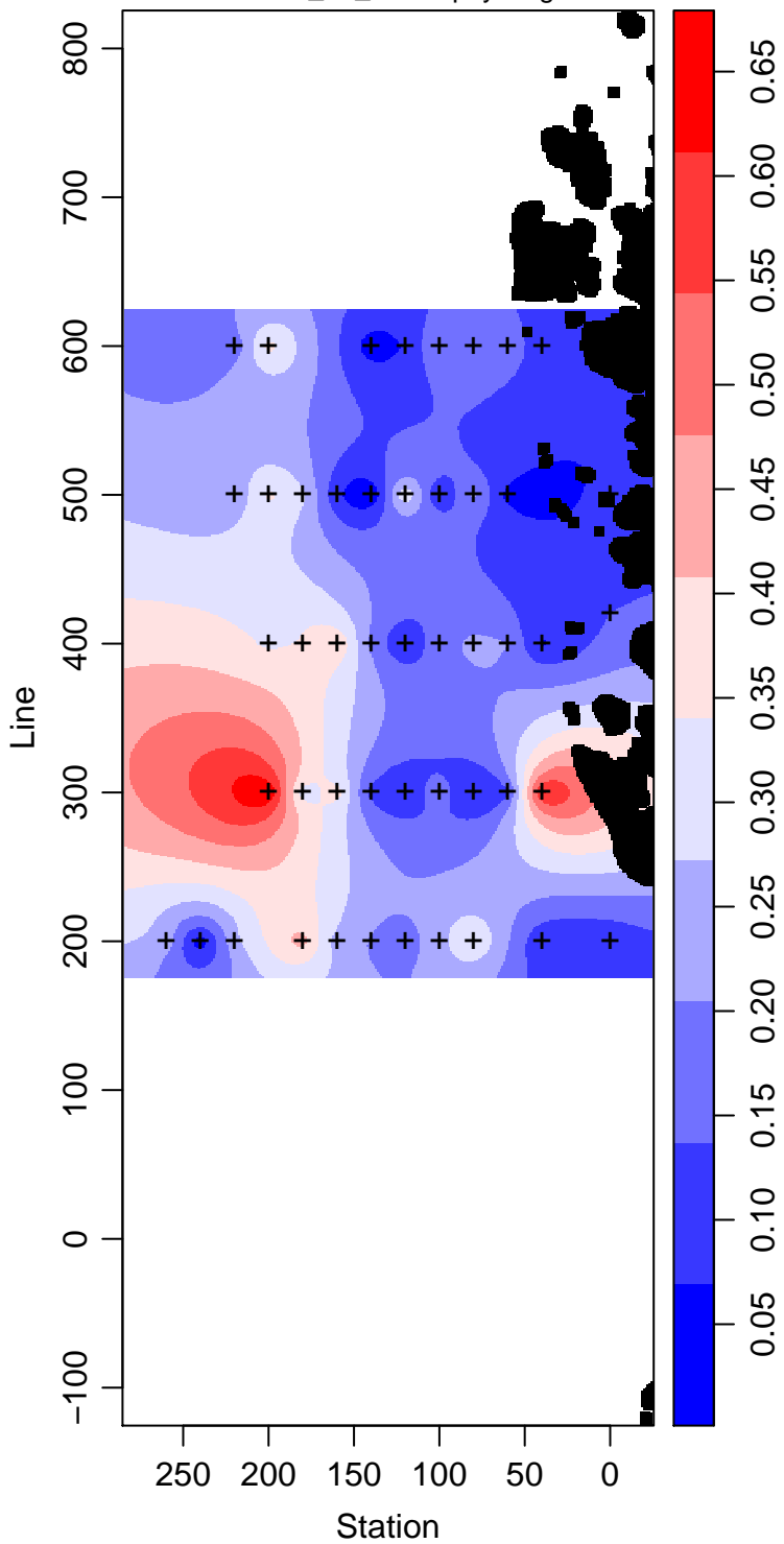
LMG08-01_80_Chlorophyll mg m -3
