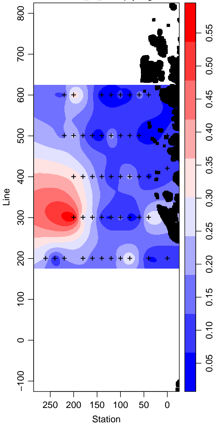
LMG08-01_90_Chlorophyll mg m -3
