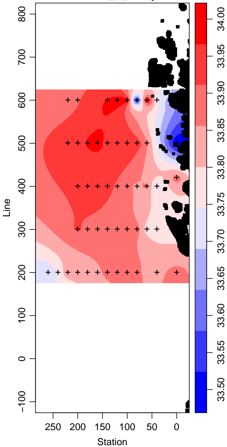
LMG08-01_10_Salinity
