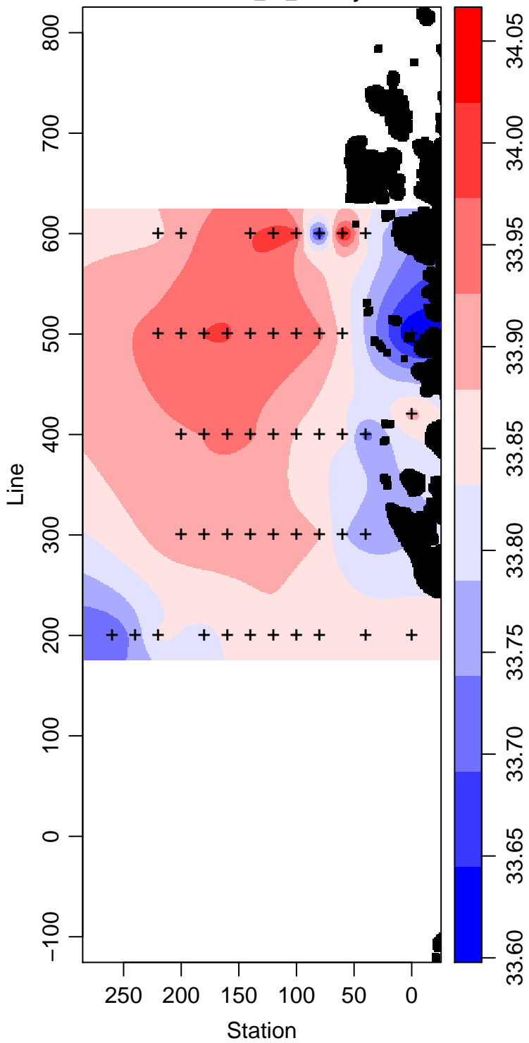
LMG08-01_15_Salinity
