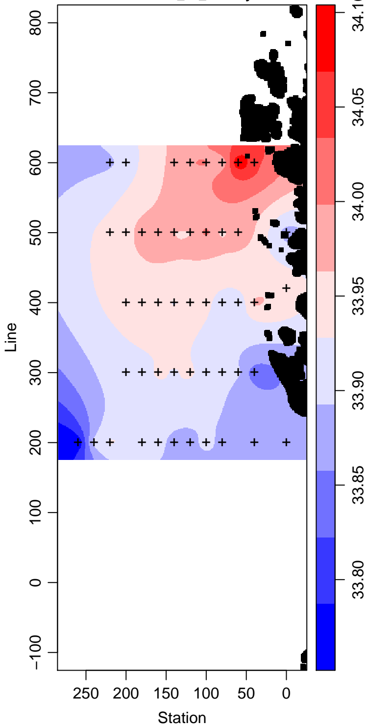
LMG08-01_40_Salinity
