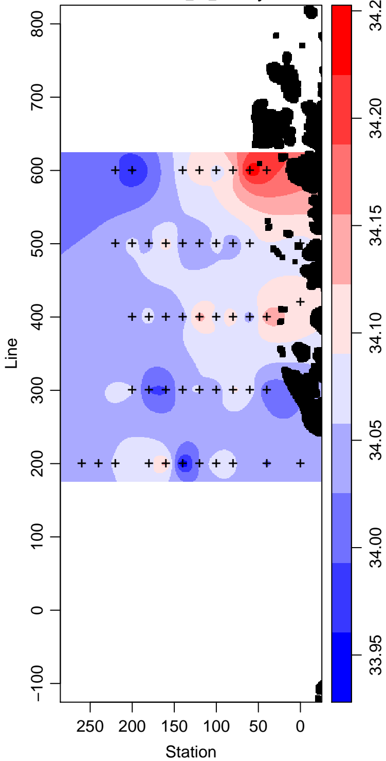
LMG08-01_75_Salinity
