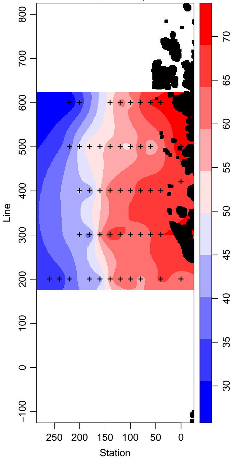
LMG08-01_35_Silicate \mu\text{ mol L}^{-1}
