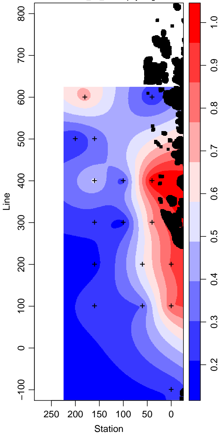
LMG09-01_50_Chlorophyll mg m -3
