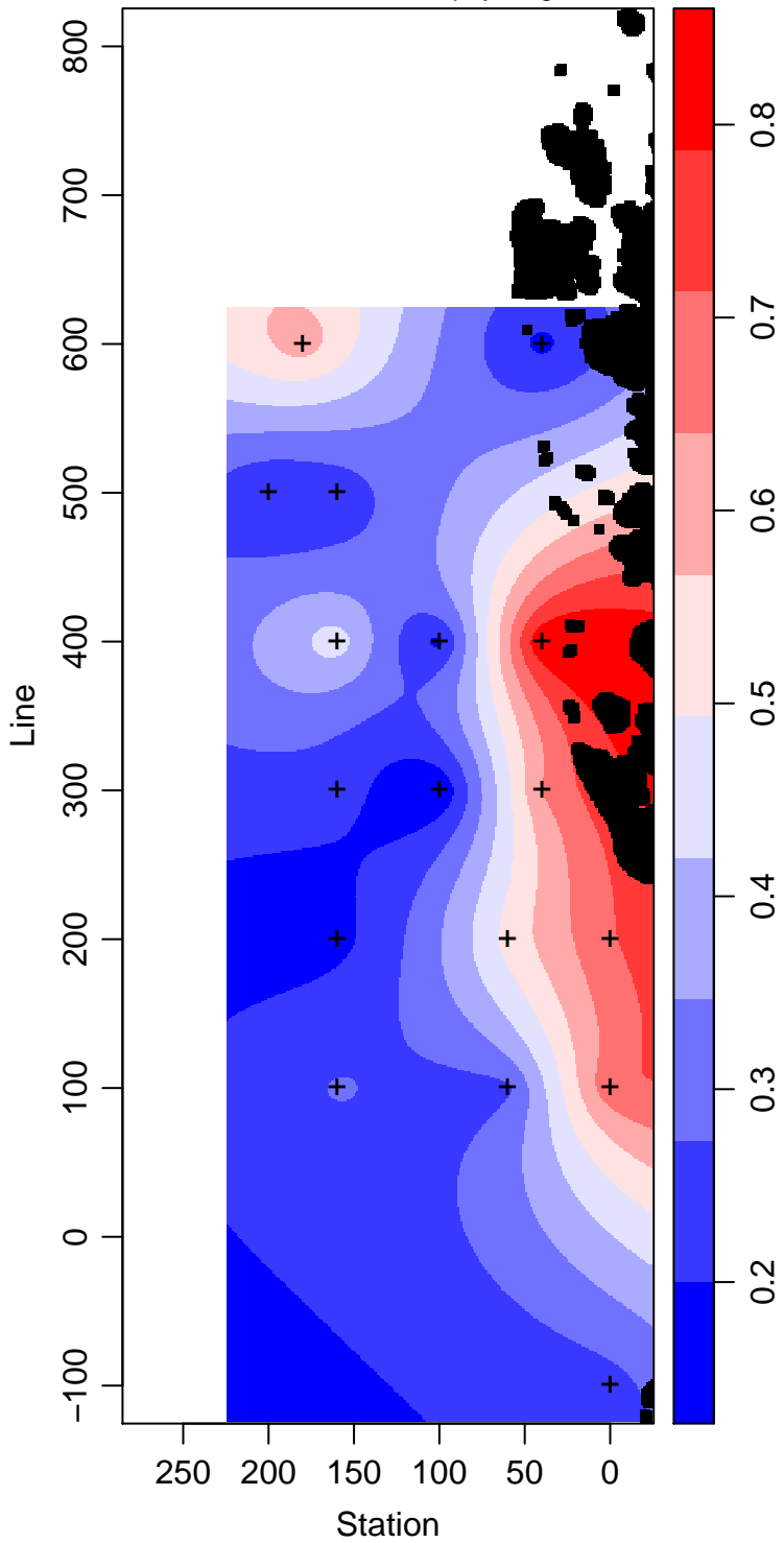
LMG09-01_55_Chlorophyll mg m -3
