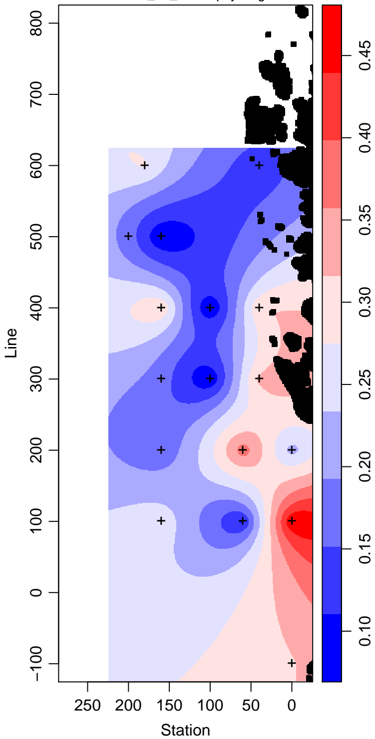
LMG09-01_70_Chlorophyll mg m -3
