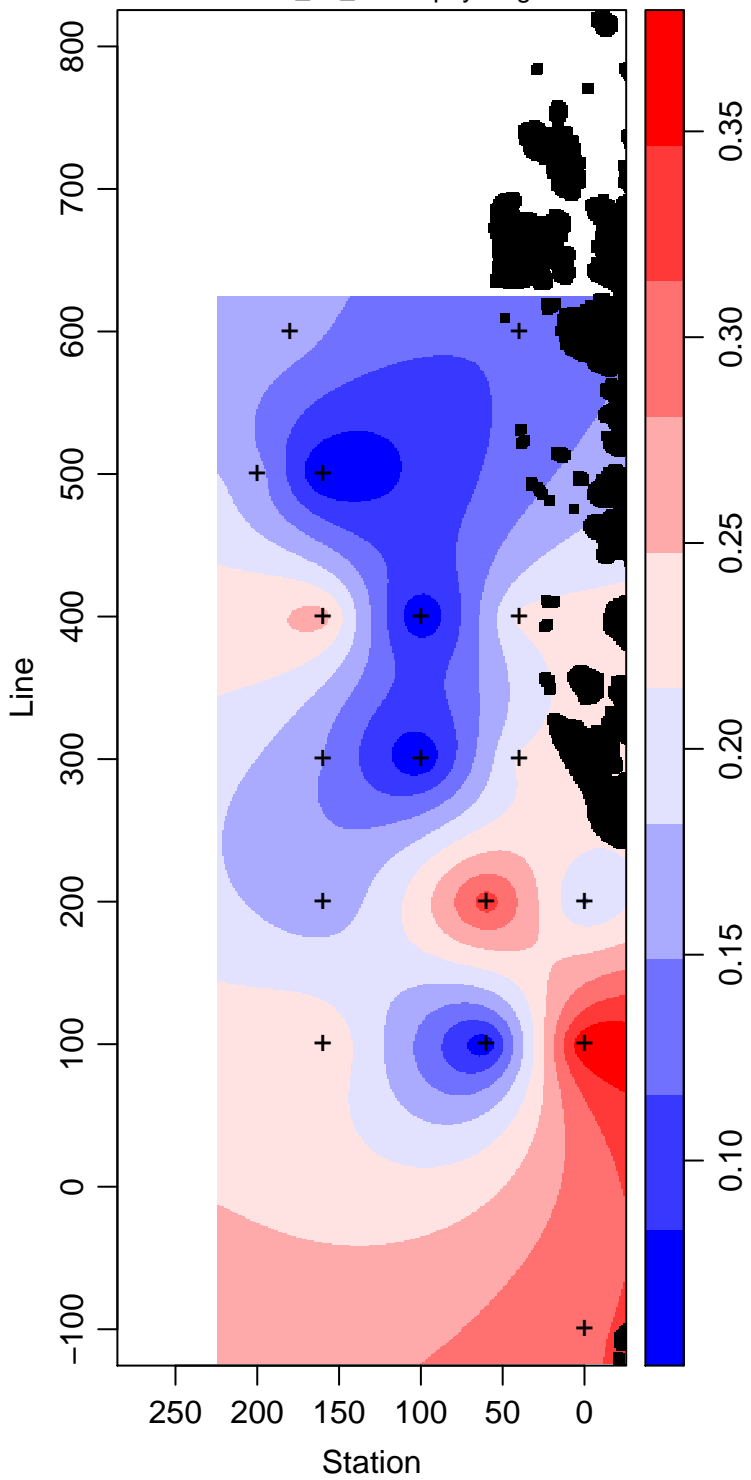
LMG09-01_75_Chlorophyll mg m -3
