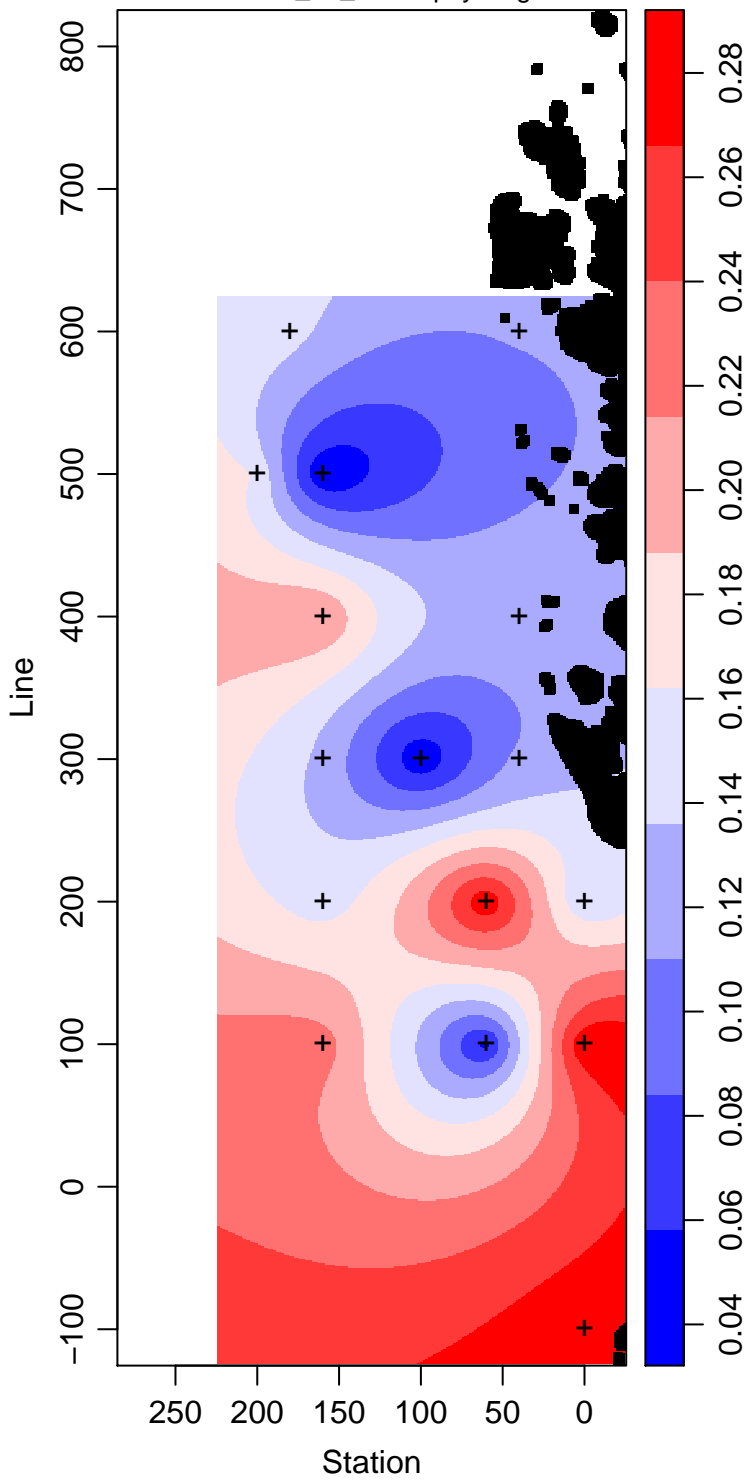
LMG09-01_80_Chlorophyll mg m -3
