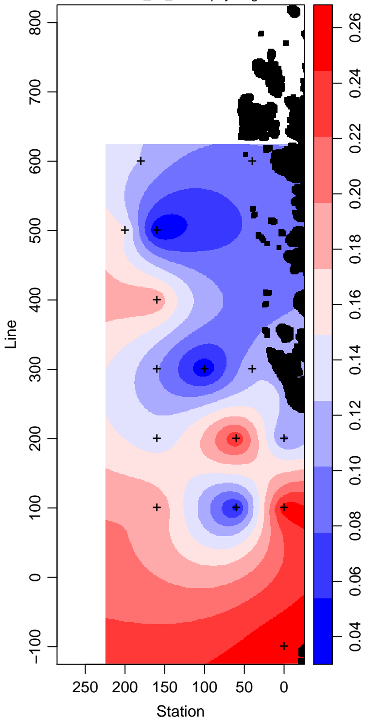
LMG09-01_85_Chlorophyll mg m -3
