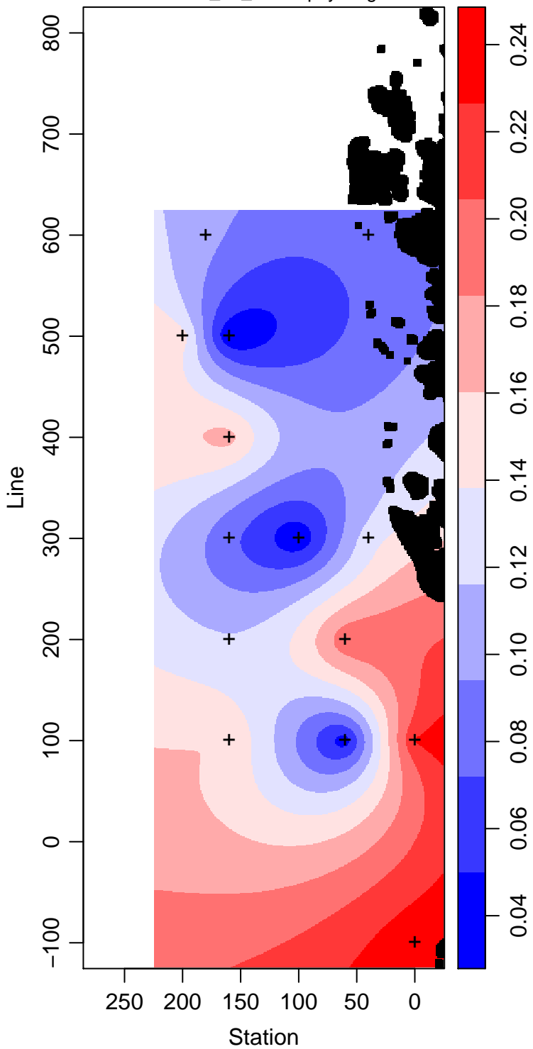
LMG09-01_90_Chlorophyll mg m -3
