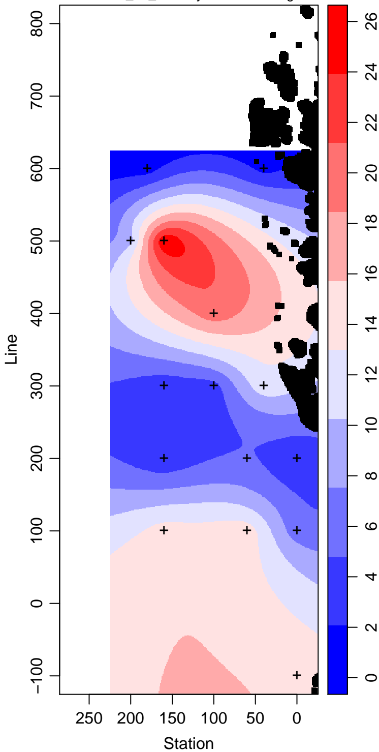
LMG09-01_35_Primary.Production mg m -3
