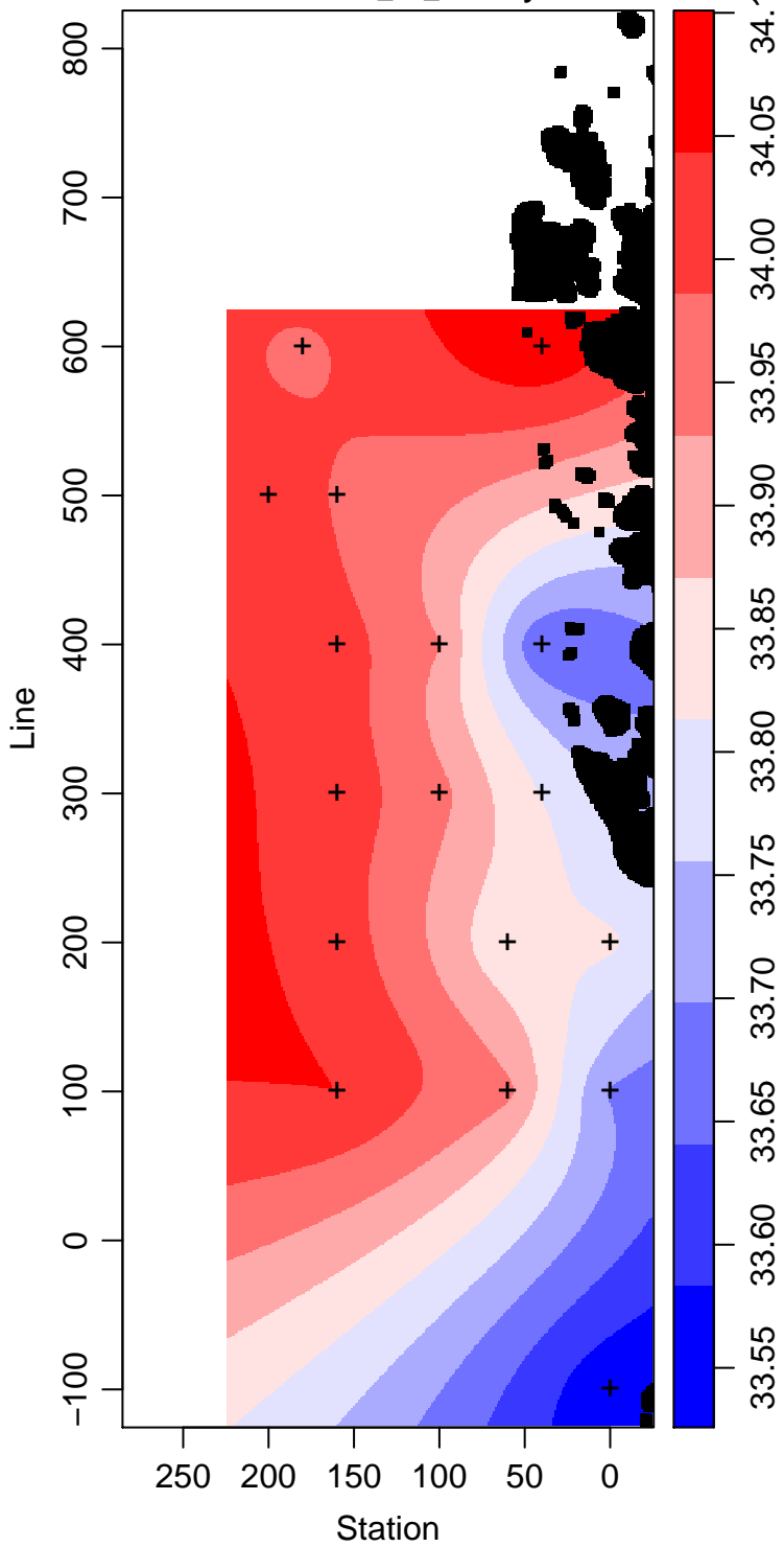
LMG09-01_40_Salinity
