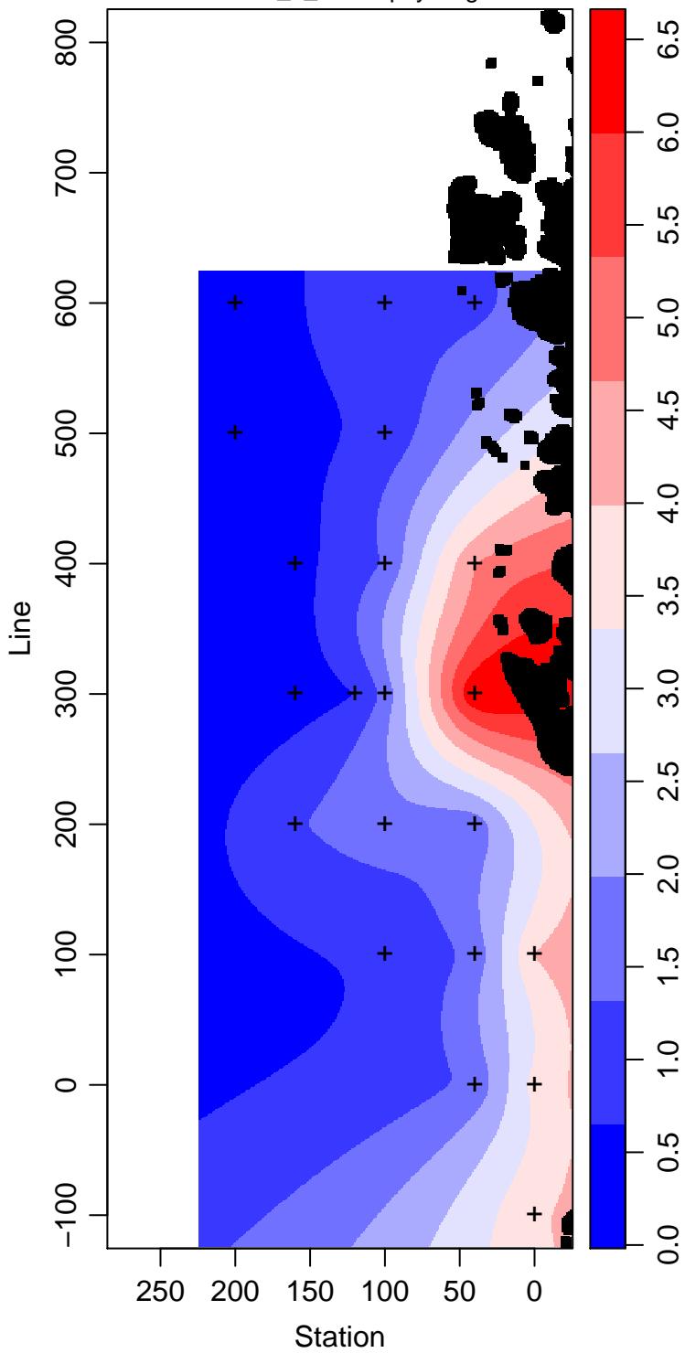
LMG10-01_1_Chlorophyll mg m -3
