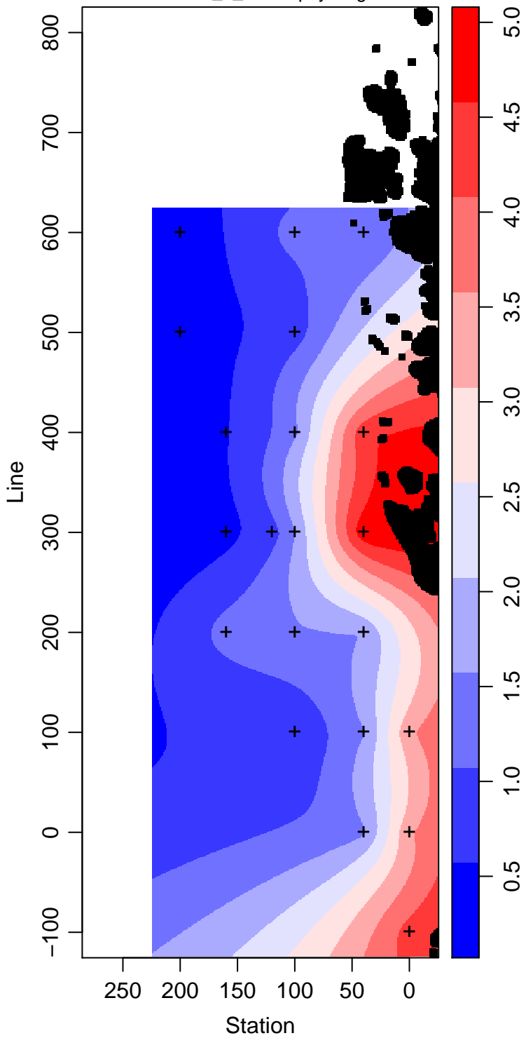
LMG10-01_5_Chlorophyll mg m -3
