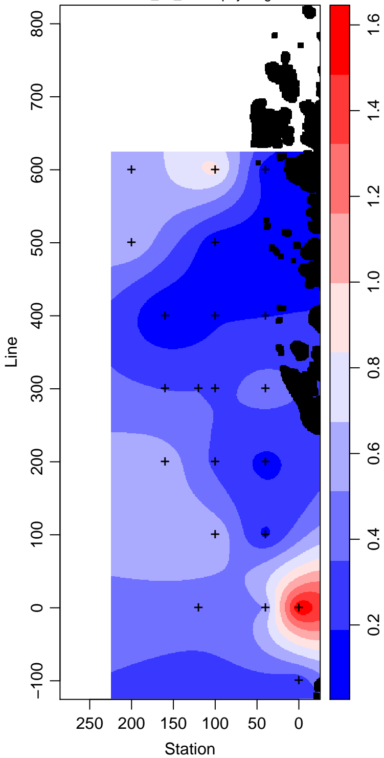
LMG10-01_75_Chlorophyll mg m -3
