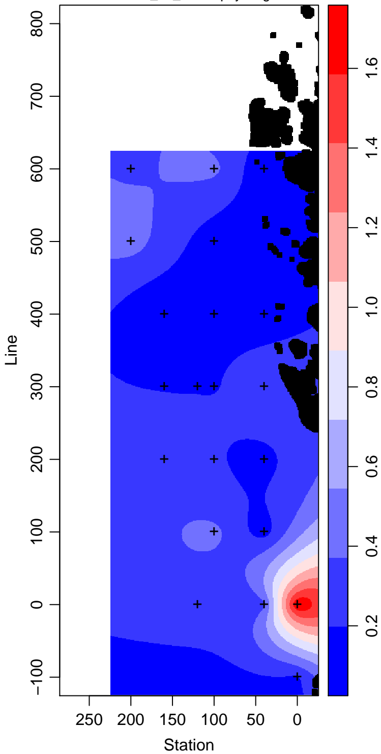
LMG10-01_90_Chlorophyll mg m -3
