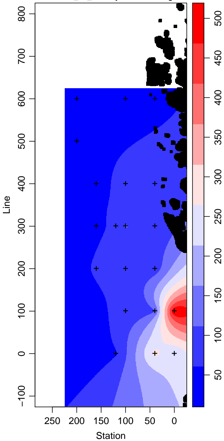
LMG10-01_40_Primary.Production mg m -3
