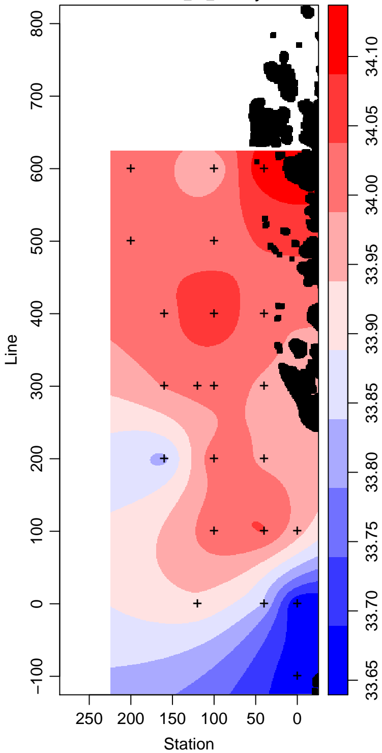
LMG10-01_70_Salinity
