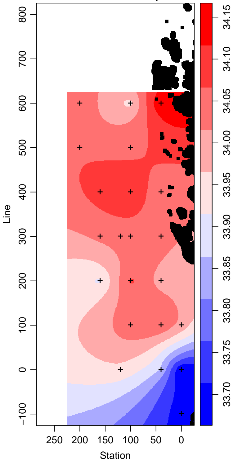
LMG10-01_75_Salinity
