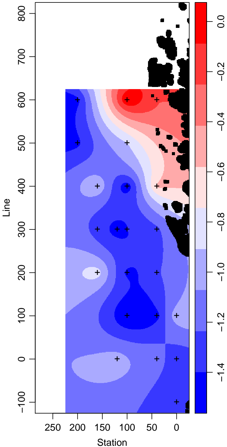
LMG10-01_70_Temperature ° Celsius
