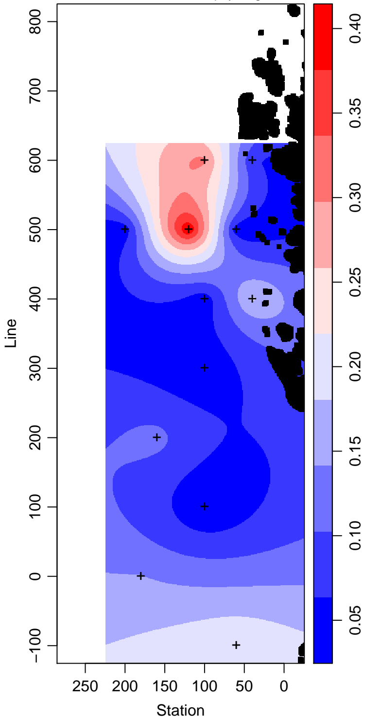
LMG11-01_100_Chlorophyll \text{mg m}^{-3}
