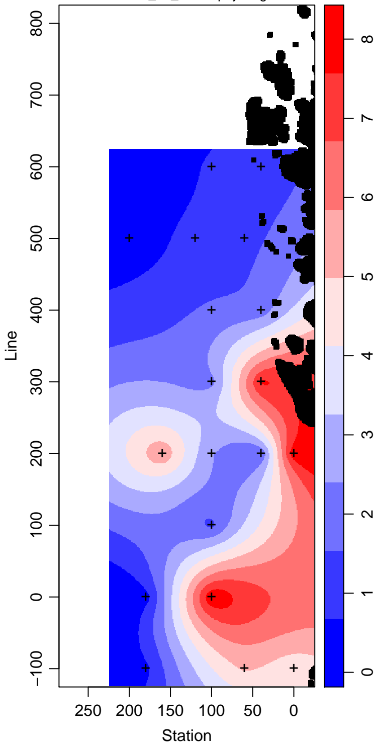
LMG11-01_10_Chlorophyll mg m -3
