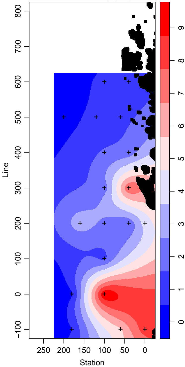
LMG11-01_15_Chlorophyll mg m -3
