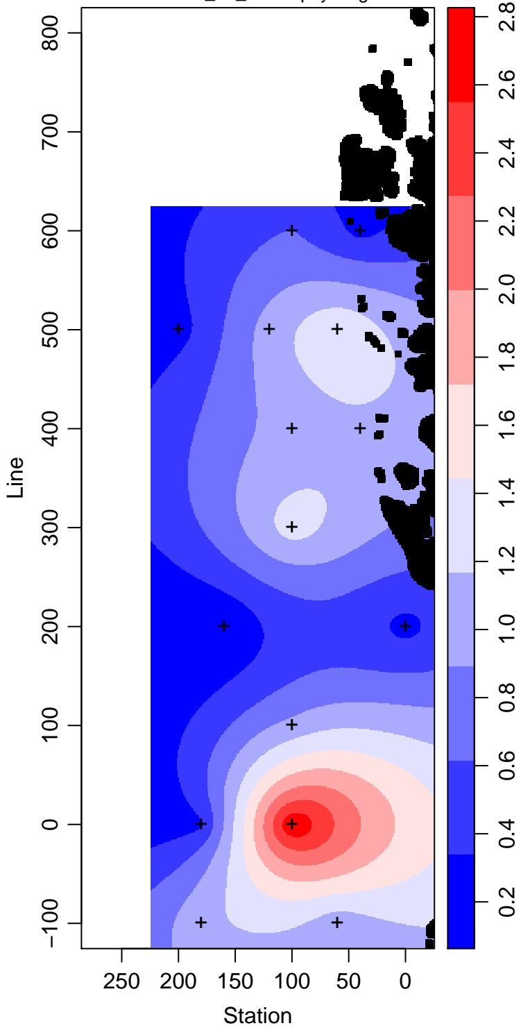
LMG11-01_45_Chlorophyll mg m -3
