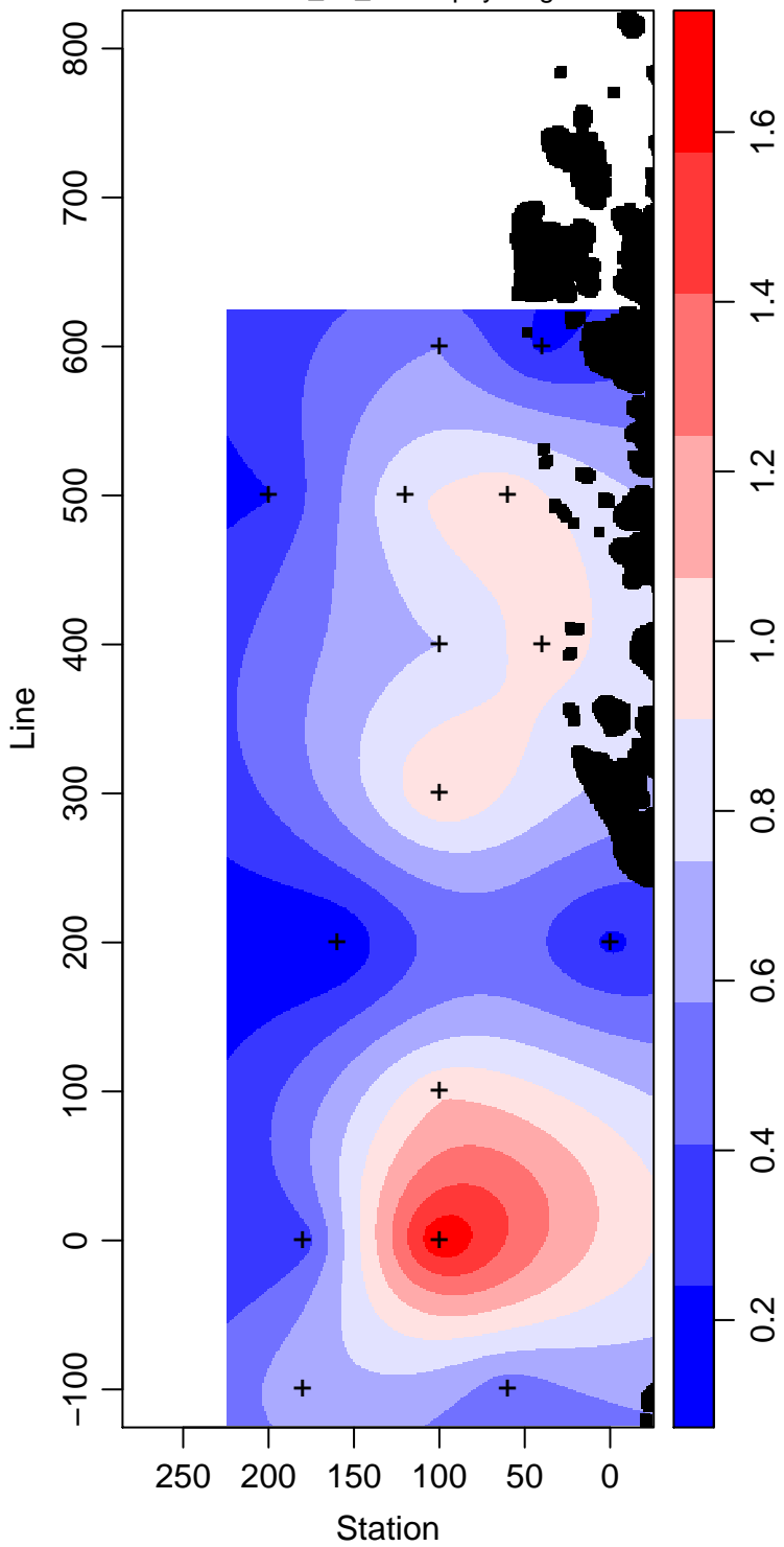
LMG11-01_55_Chlorophyll mg m -3
