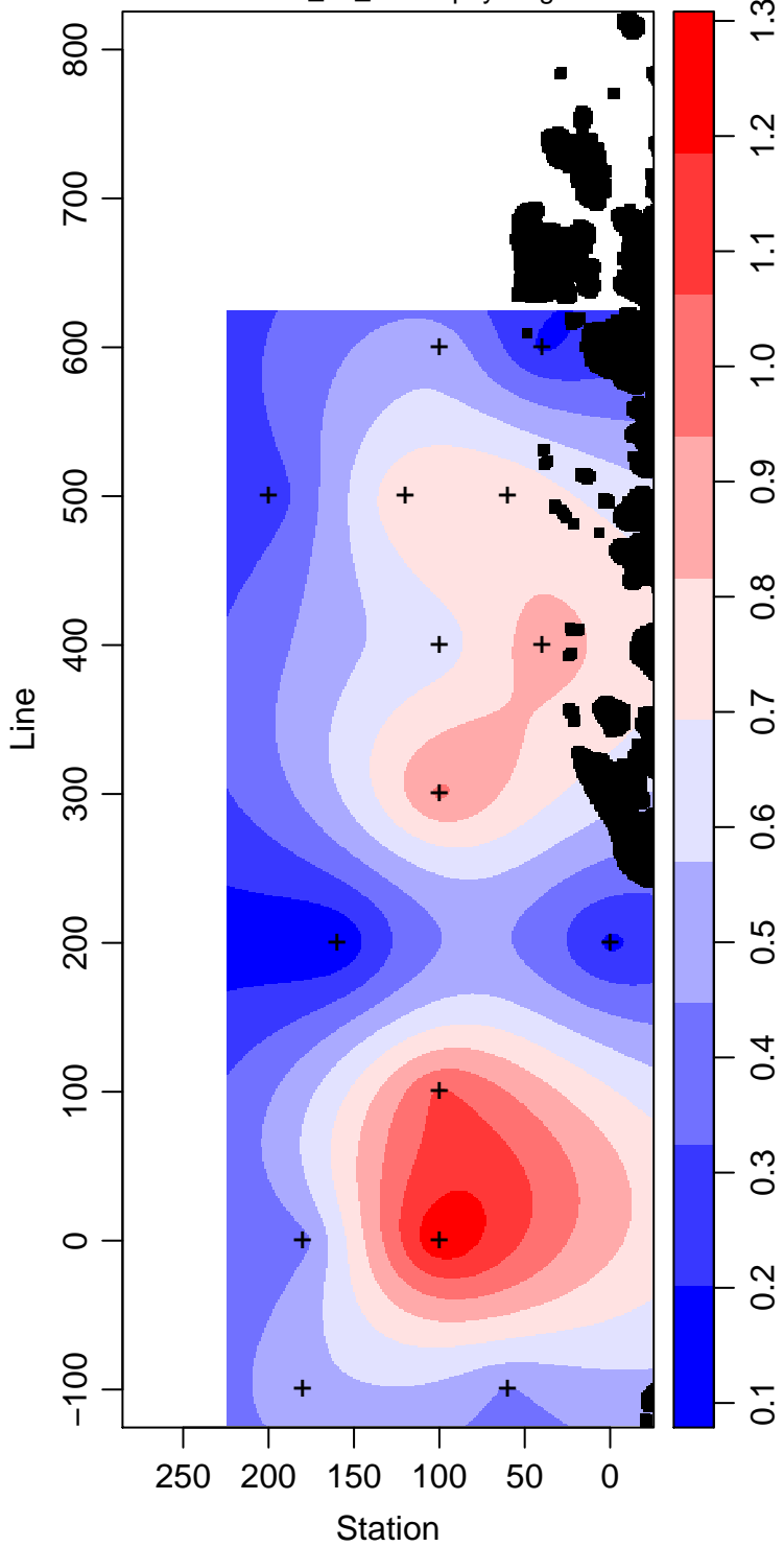
LMG11-01_60_Chlorophyll mg m -3
