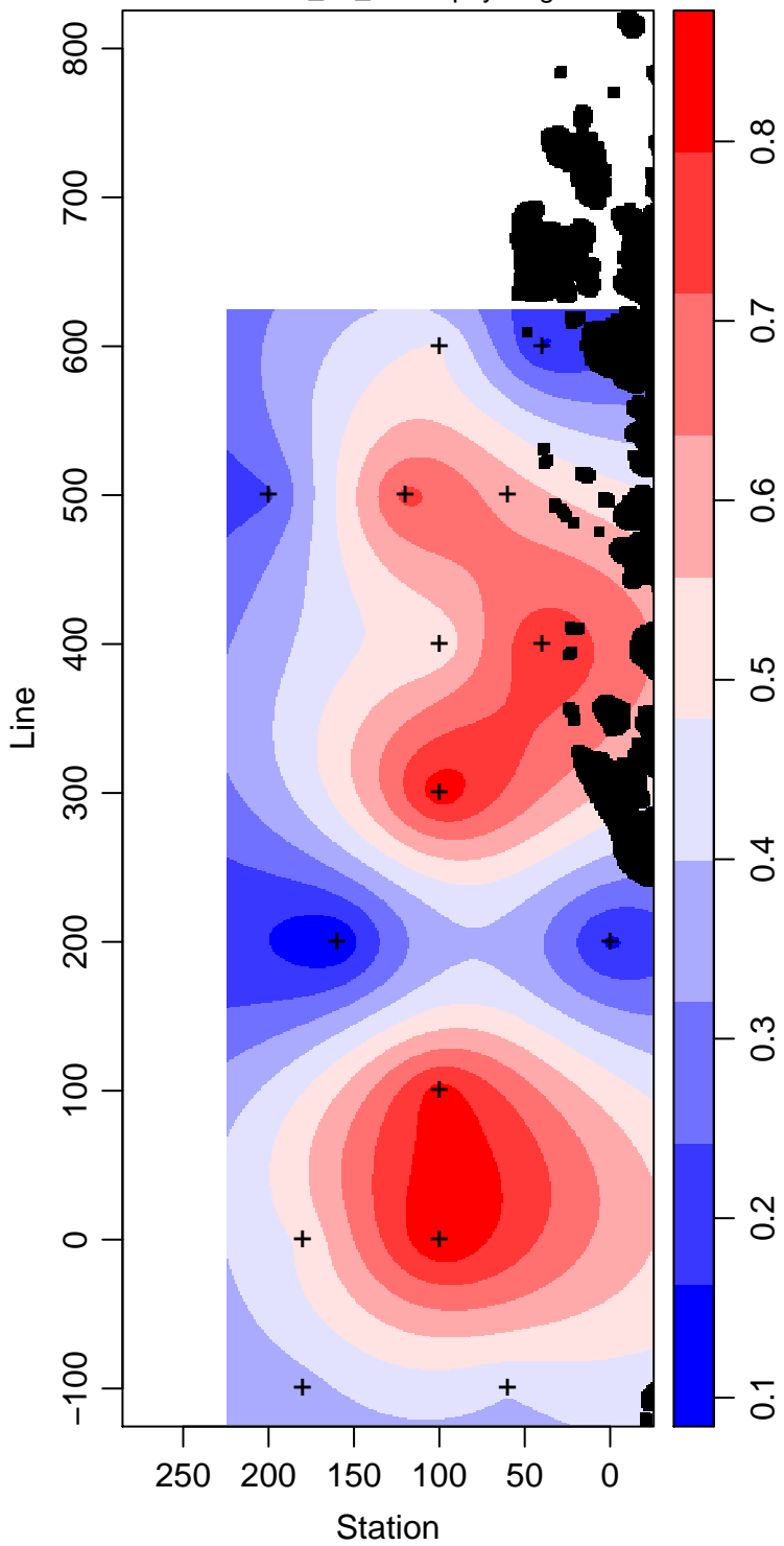
LMG11-01_65_Chlorophyll mg m -3
