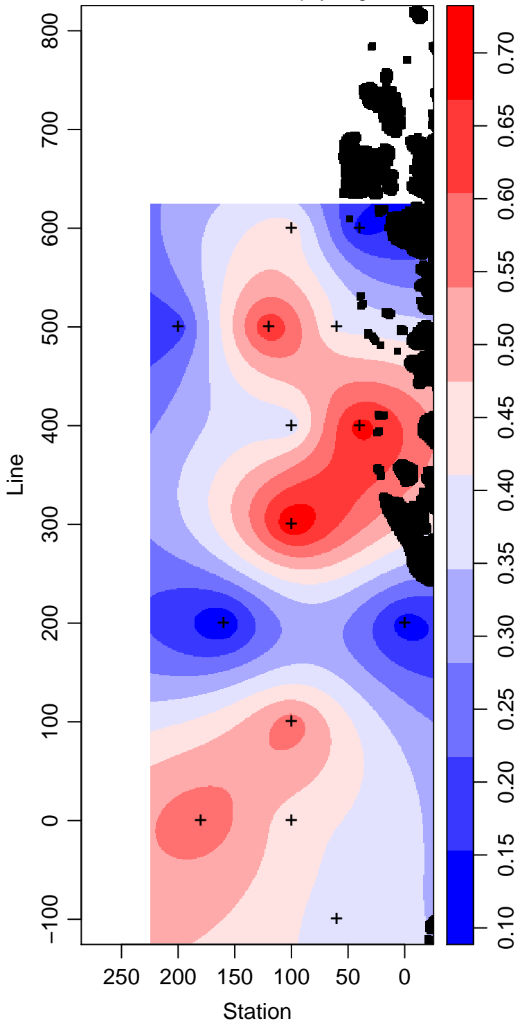
LMG11-01_70_Chlorophyll mg m -3
