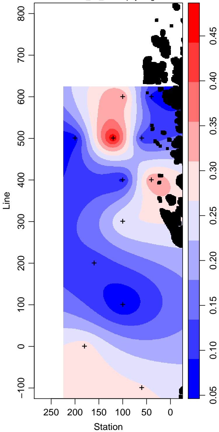
LMG11-01_90_Chlorophyll mg m -3
