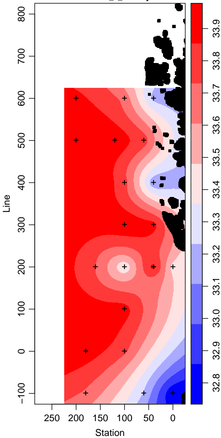
LMG11-01_1_Salinity
