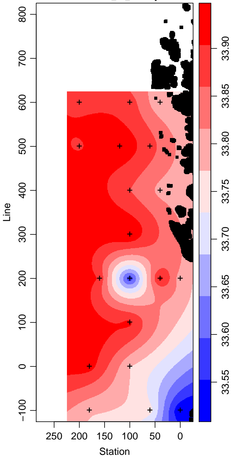
LMG11-01_35_Salinity
