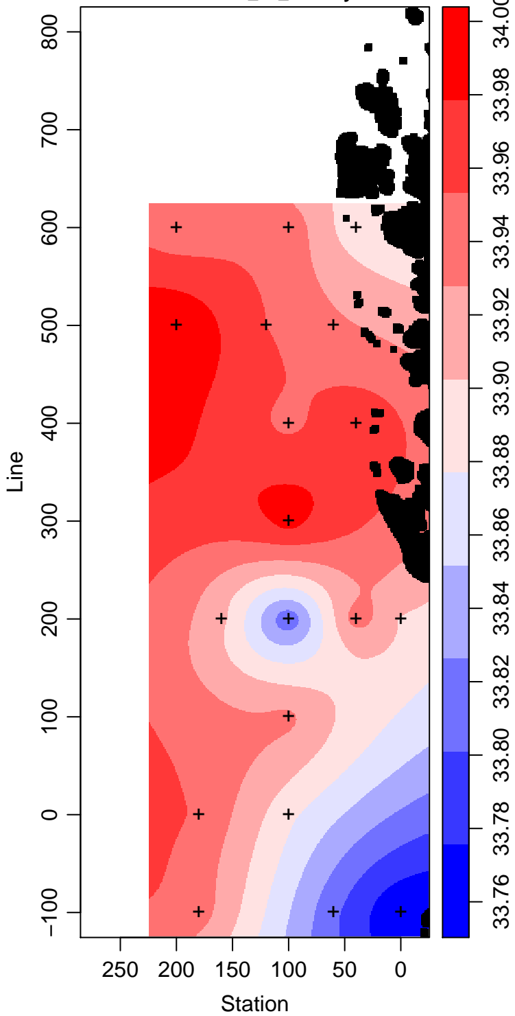
LMG11-01_65_Salinity
