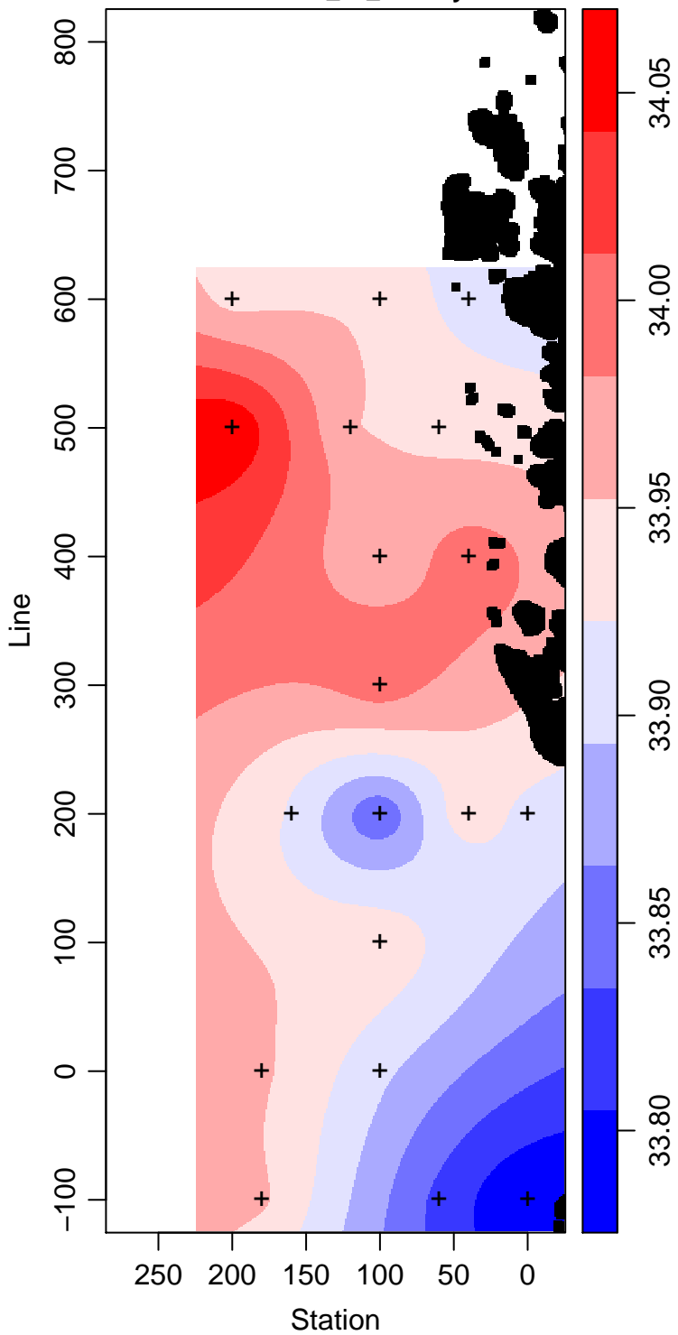
LMG11-01_70_Salinity
