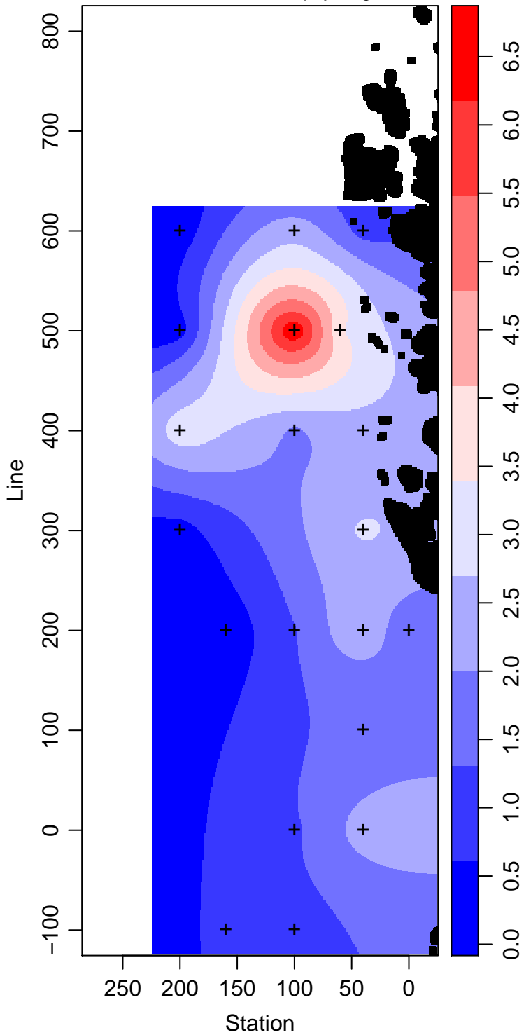
LMG12-01_15_Chlorophyll mg m -3
