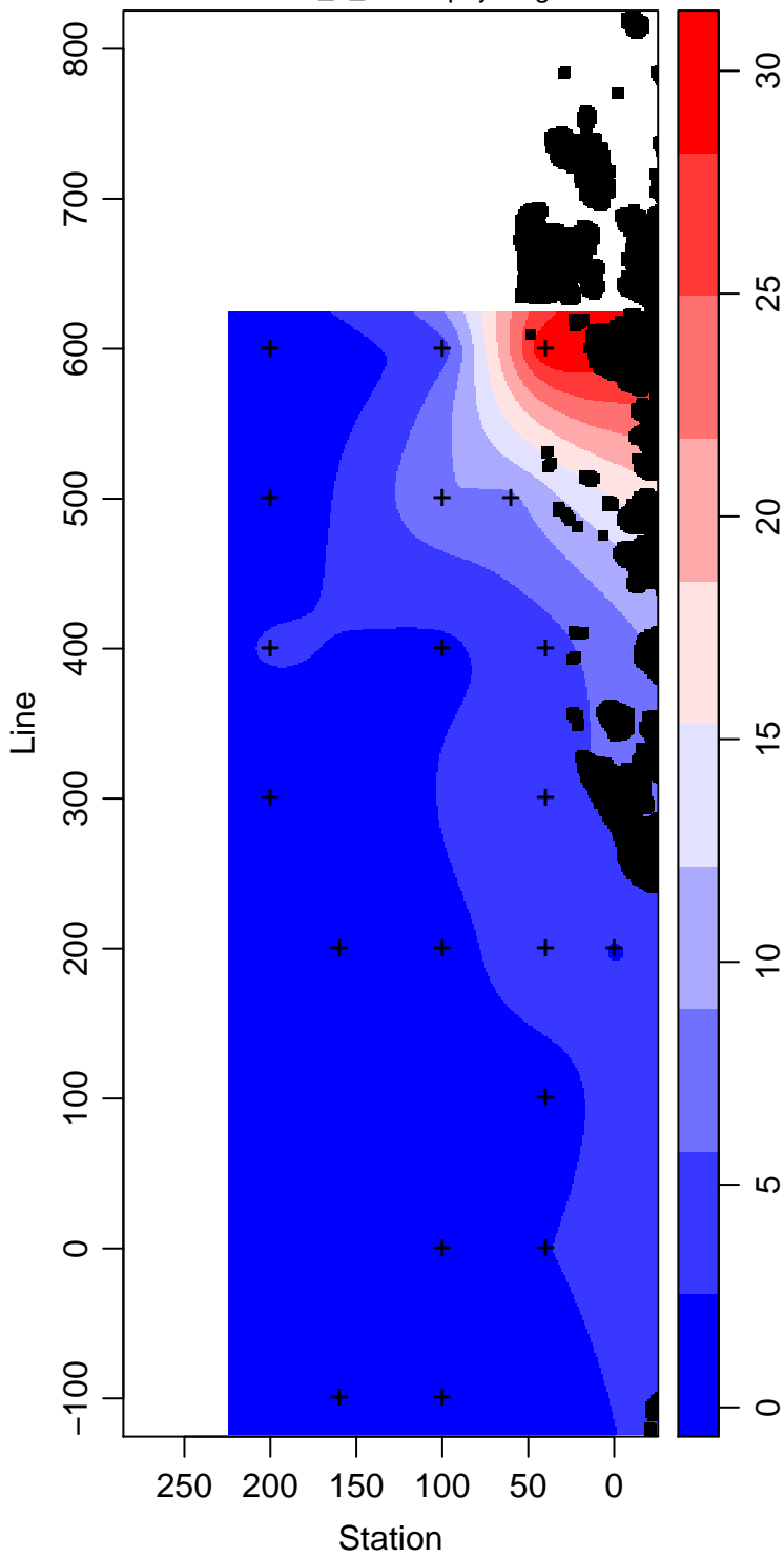
LMG12-01_5_Chlorophyll mg m -3
