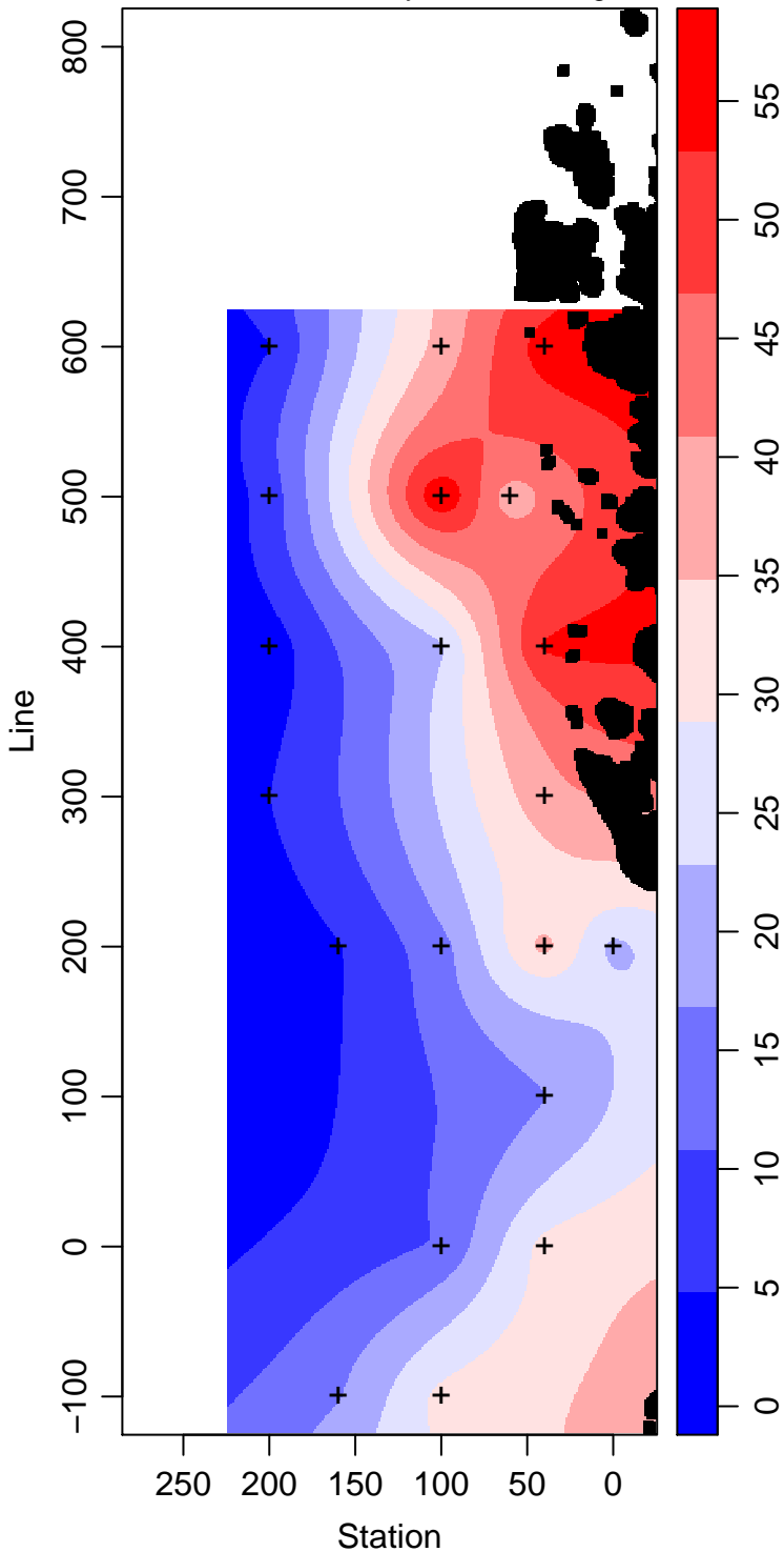
LMG12-01_10_Primary.Production mg m -3
