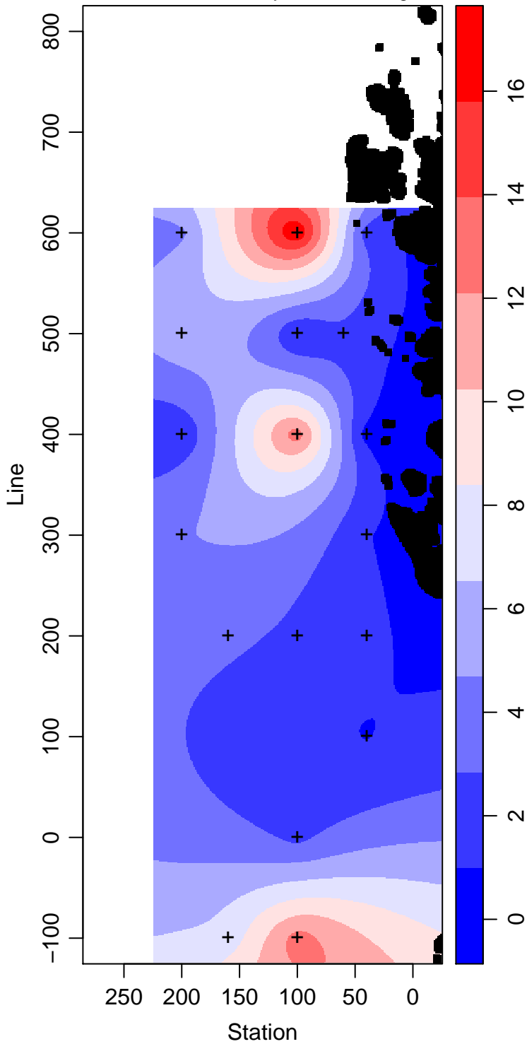
LMG12-01_35_Primary.Production mg m -3
