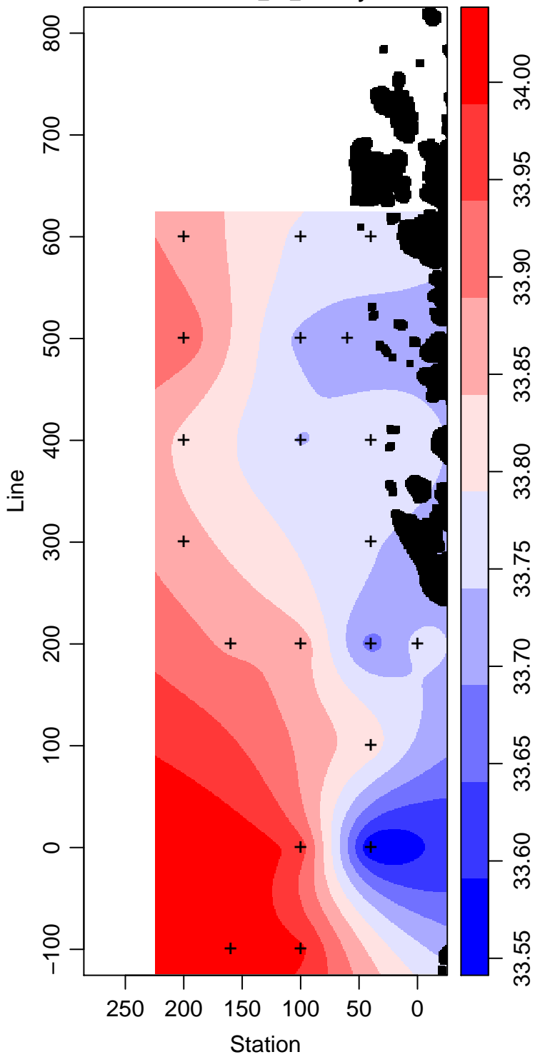
LMG12-01_35_Salinity
