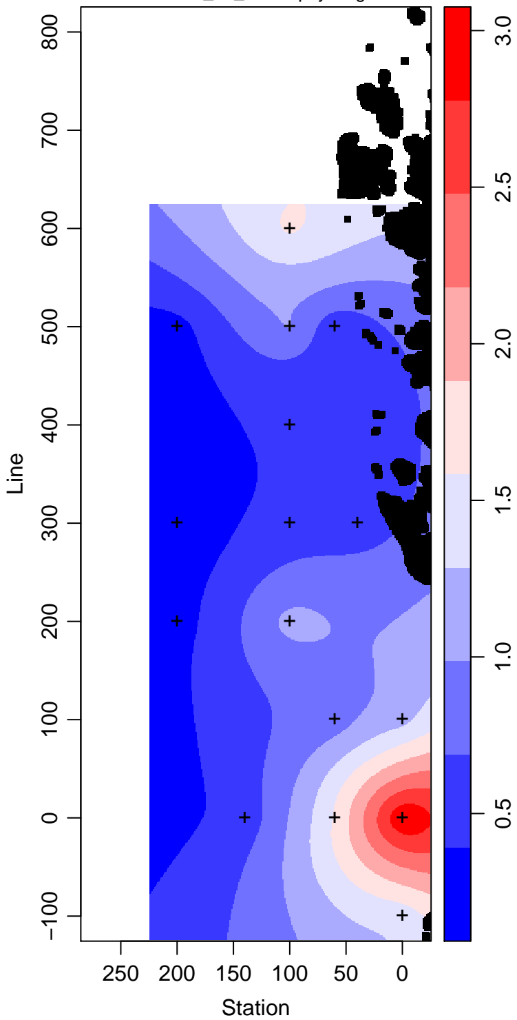
LMG13-01_15_Chlorophyll mg m -3
