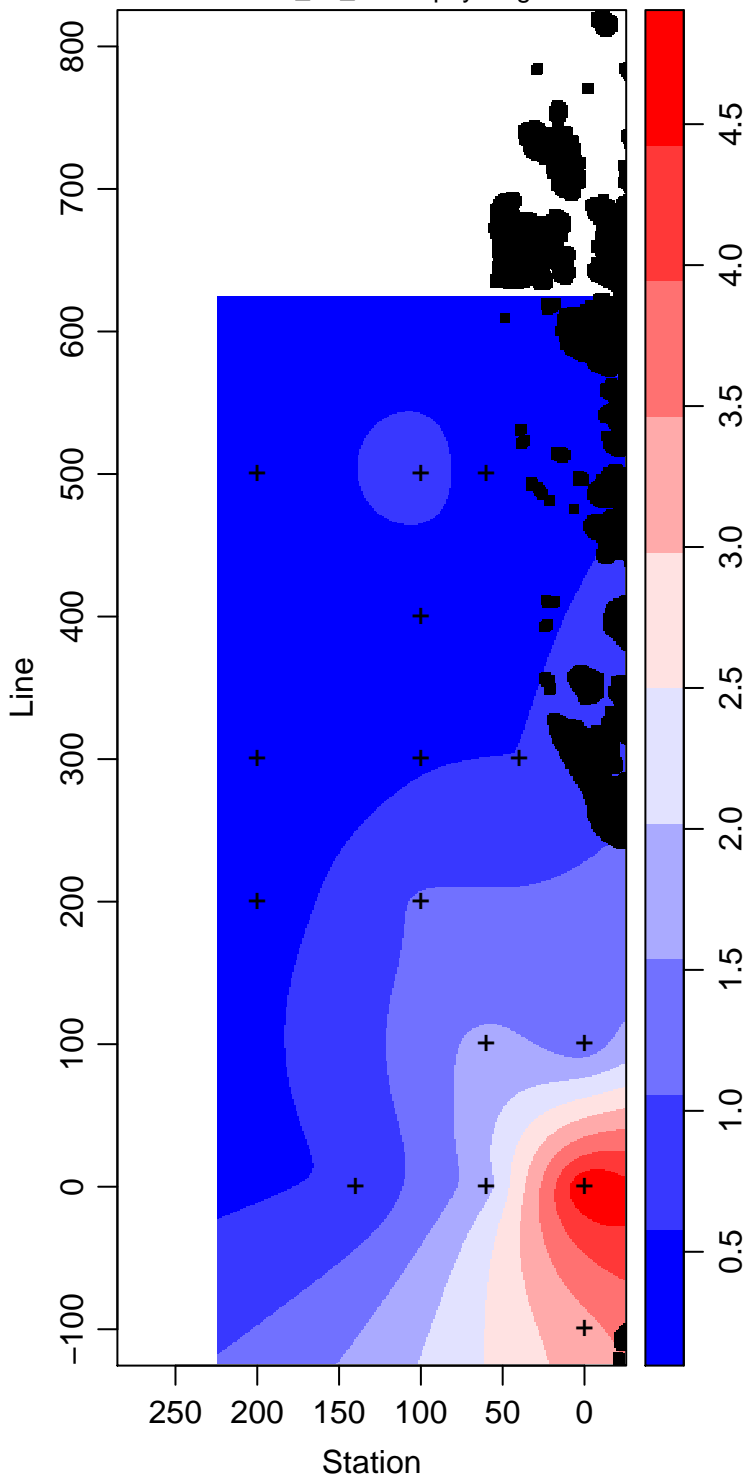
LMG13-01_25_Chlorophyll mg m -3
