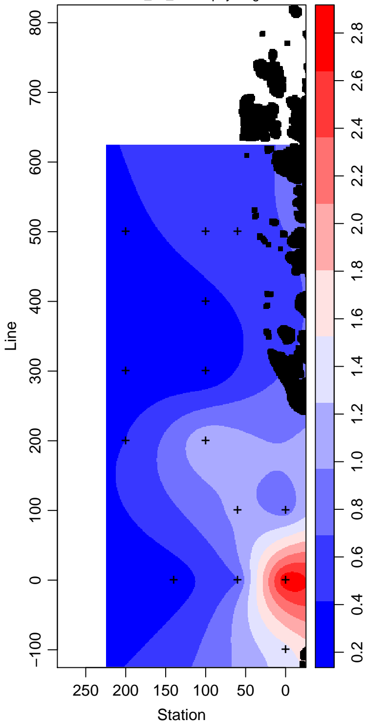
LMG13-01_45_Chlorophyll mg m -3
